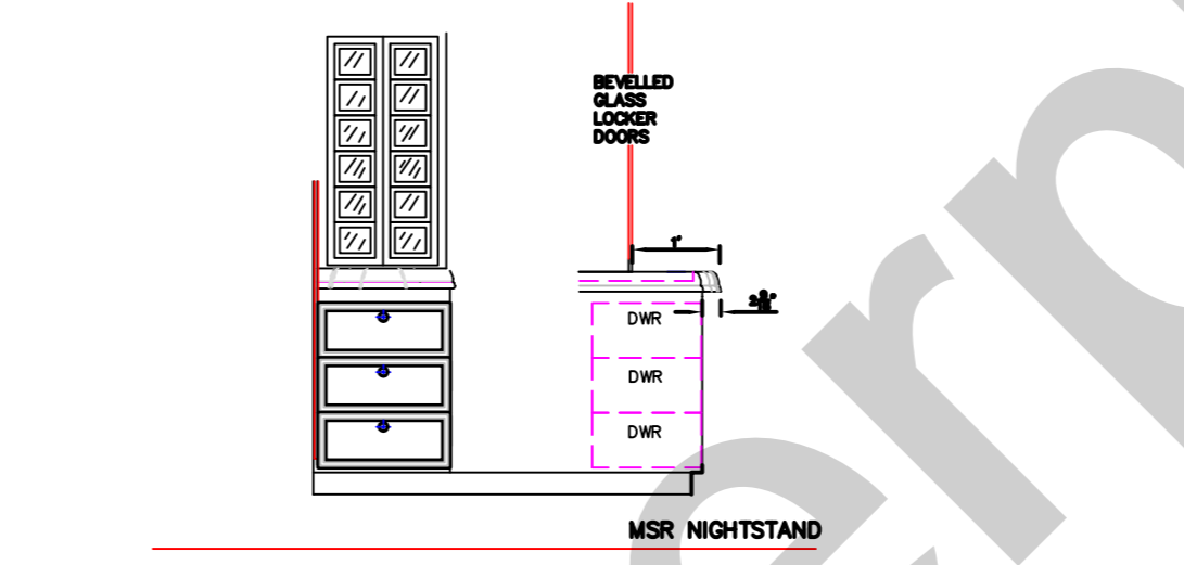
MSR NIGHTSTAND 1/2"=1'-0"
